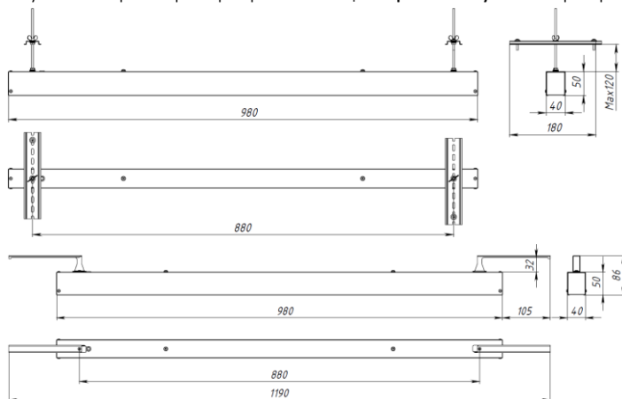
Рисунок 4 - Габаритные размеры при комплектации с креплением для реечного потолка на примере Line 980мм.
