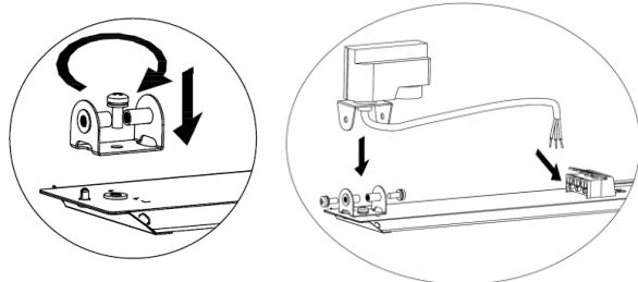
Рисунок 9. Установка крепления с адаптером для 1-фазного шинпровода и подключение.
