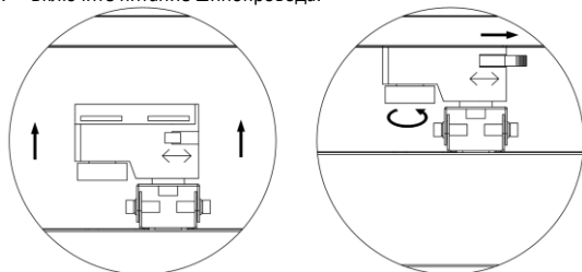
Рисунок 10. Крепление на шинпроводе.
