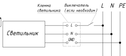
Рисунок 5. Схема подключения светильника.
